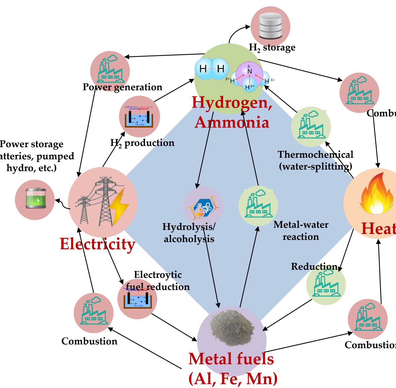
カーボンフリー二次エネルギー間の関係
