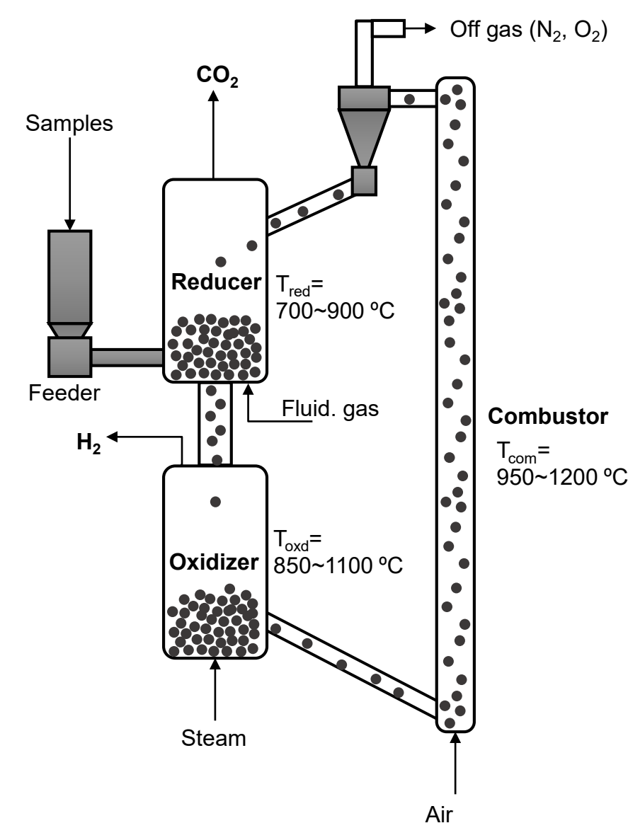
CO 2 フリーケミカルルーピング水素製造システム
