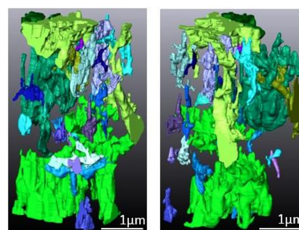
FIB-SEMによる空隙構造観察
