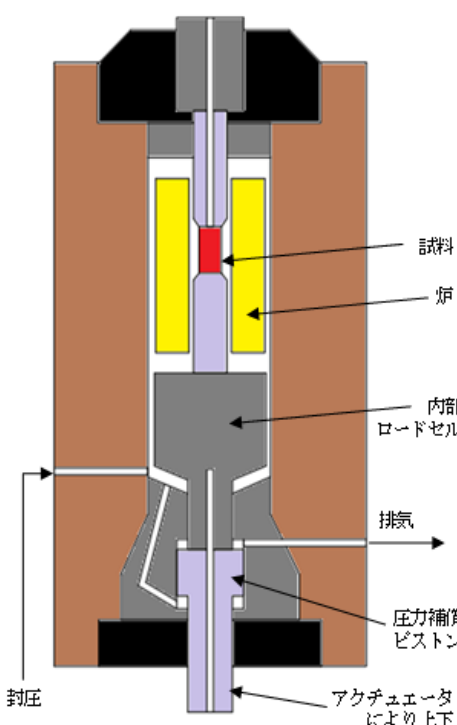
高圧三軸試験装置 (Brown Univ.)
