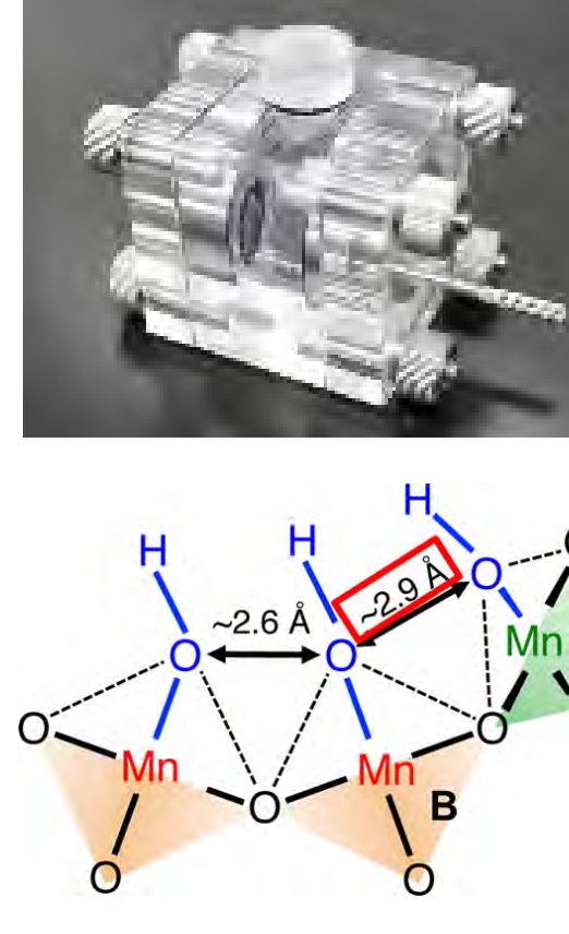
試作した金属-空気電池
