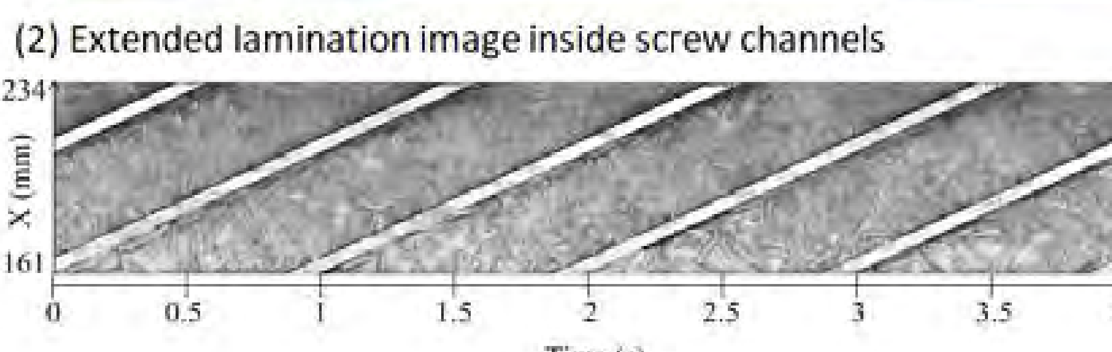
長繊維強化樹脂可塑化過程の可視化解析
